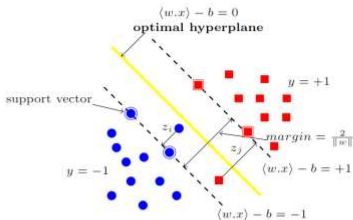
Hình 5. Phân lớp tuyến tính với máy học SVM
